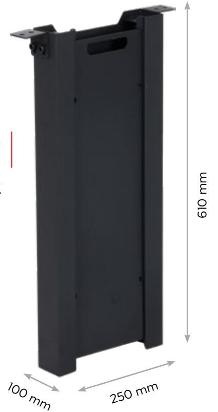
ORTA DESTEK & KABLO KANALI CENTER COLUMN & CABLE SOCKET
